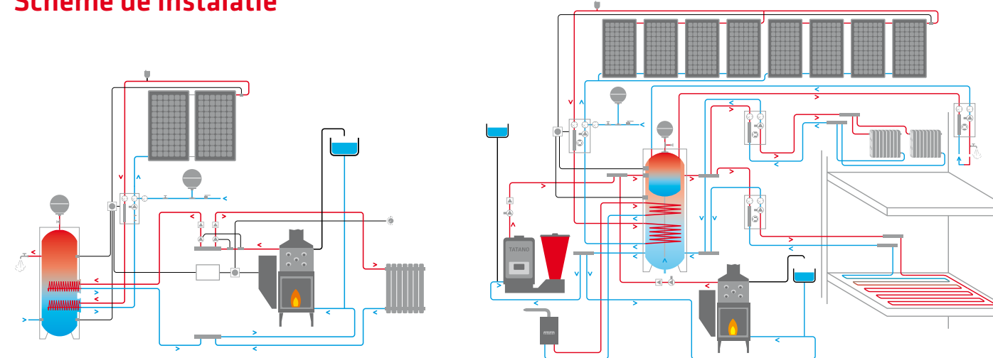
Sistem solar centralizat fortat, integrat de termo-semineu
